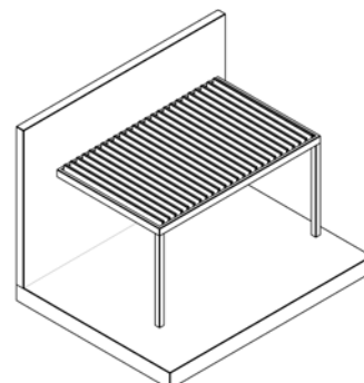
TYP 2 Montáž na stenu, lamely kolmé na stenu
